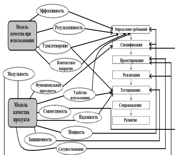
Рис. 2. Принадлежность характеристик качества этапам жизненного цикла программного обеспечения
