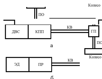
Рис. 1. Функциональные схемы трансмиссий автомобиля (а) и электромотоцикла (б)
