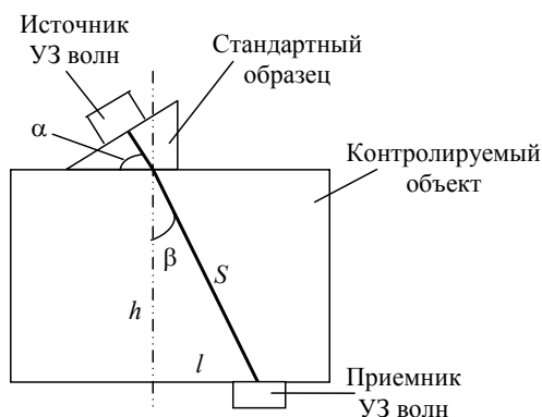
Схема ультразвукового прозвучивания образца из синтегрона
