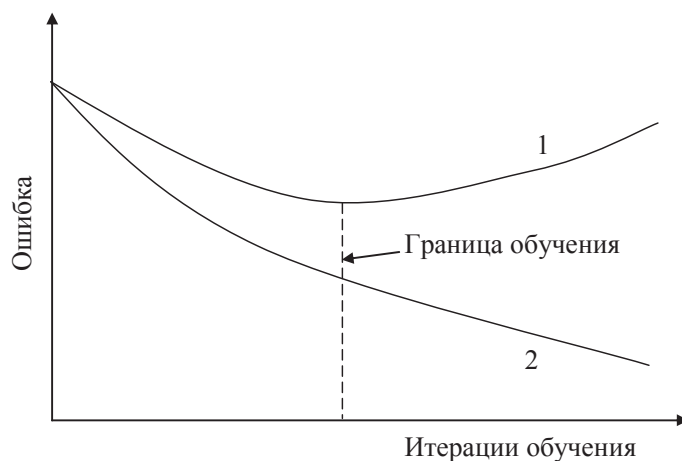
1 – ошибка на тестовом множестве обучающей выборки 2 – ошибка на обучающем множестве обучающей выборки
