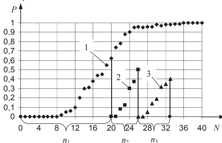
Рис. 3 – «Облака» точек при испытаниях НС без повторного обучения (1) и с повторным обучением (2)
