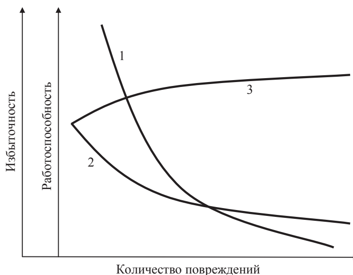
Рис. 2 – Влияние количества повреждений на уменьшение избыточности (1) и падение работоспособности не подвергающихся (2) и подвергающихся повторному обучению (3) НС
